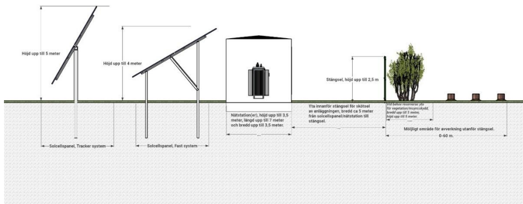
Figur 19. Principskiss över utformning av solpark i skogsmark. Tillkommer gör även internt el och vägnät, uppställningsytor och eventuell energilagringenshet.
